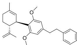
C-0111 1,3-Dimethoxy-2-((1R,6R)-3-methyl-6-(prop-1-en-2-yl)cyclohex-2-enyl)-5-phenethyl-benzene C 26 H 32 O 2 ; F.W: 376.53
